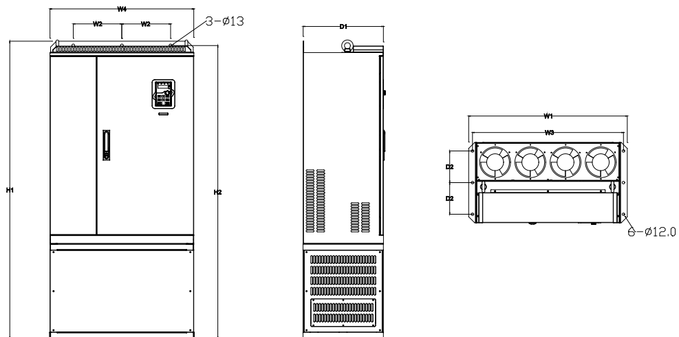
Рис. 4.13 Напольный монтаж 220 – 315 кВт
