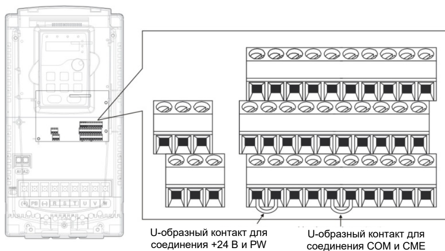
Рис.5-18 U-образный контакт
