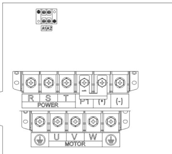
Рис. 5-10 Клеммы силовых цепей 75 – 110 кВт
