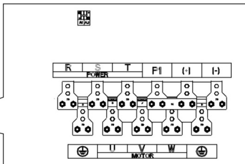
Рис. 5-11 Клеммы силовых цепей 132 – 200 кВт
