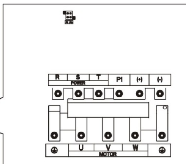
Рис. 5-11 Клеммы силовых цепей 132 – 200 кВт
