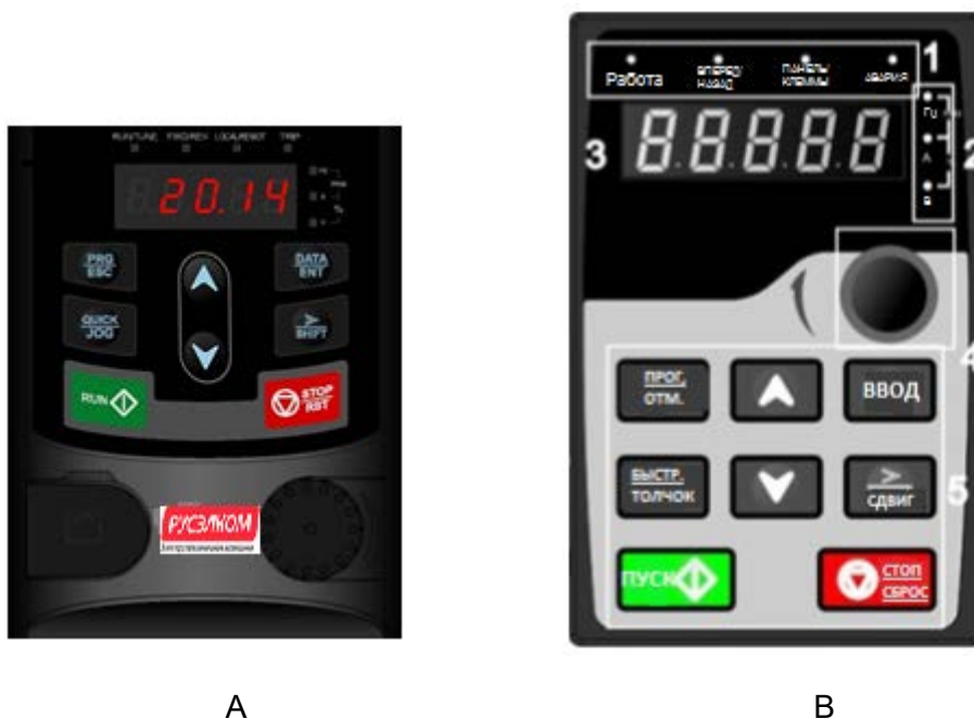
Рис. 6-1 Панель управления
