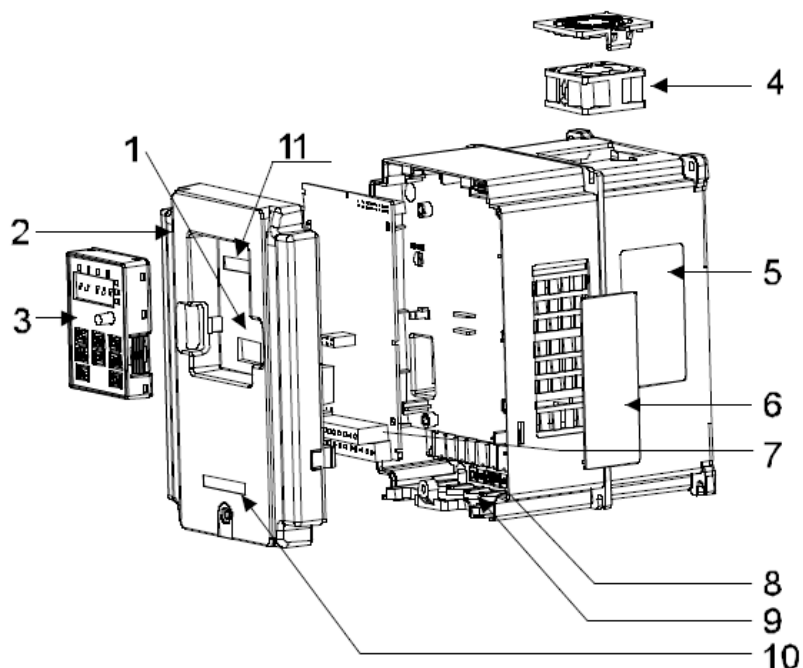
Рисунок 3-2. Структурная схема преобразователя частоты GD20 (мощностью свыше 4 кВт).
