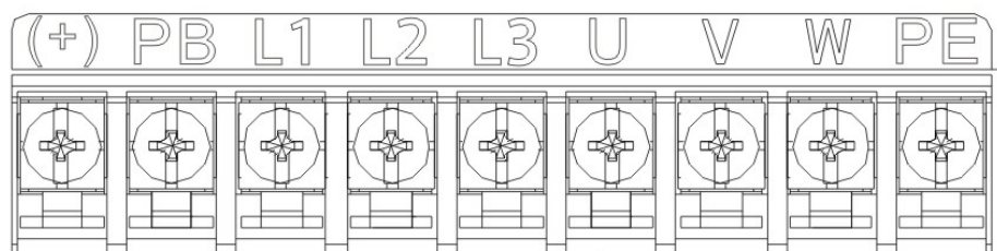
Рис. 5-5 Клеммы силовых цепей 3 фазы 380В до 2,2 кВт.
