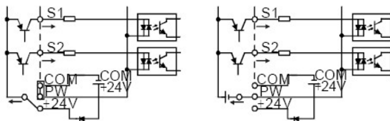
Рис.5-20 PNP режим
