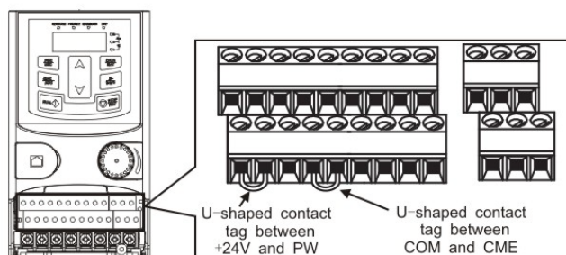
Рис.5-18 U-образный контакт
