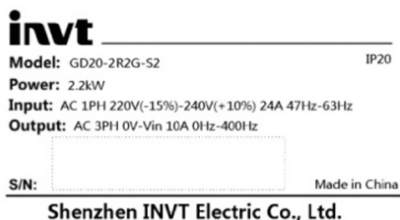
Рисунок 2-1. Шильдик преобразователей частоты GD20
