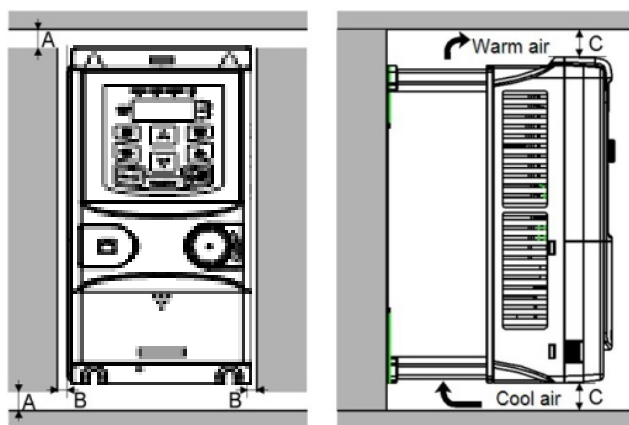
Рисунок 4-13. Вентиляционные промежутки
