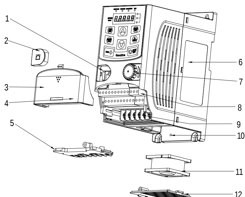
Рисунок 3-1. Структурная схема преобразователя частоты GD20.
