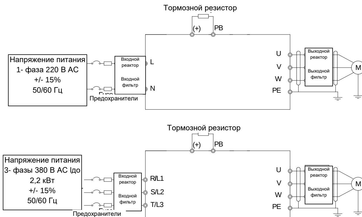
Рис. 5-3.1. Подключение силовых кабелей и управления
