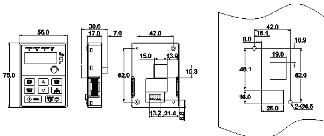
Рисунок 4-11. Внешний вид
