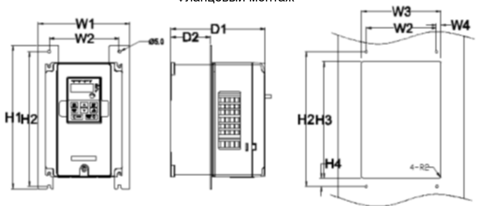
Рис. 4.10 Фланцевый монтаж 4 – 55 кВт
