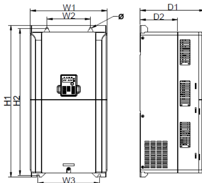
Рис. 4.8 Настенный монтаж 4 – 37 кВт
