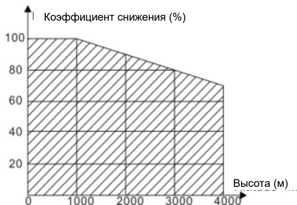
Рисунок 3-3. Снижение номинальной мощности преобразователя частоты GD20 в зависимости от высоты над уровнем моря.
