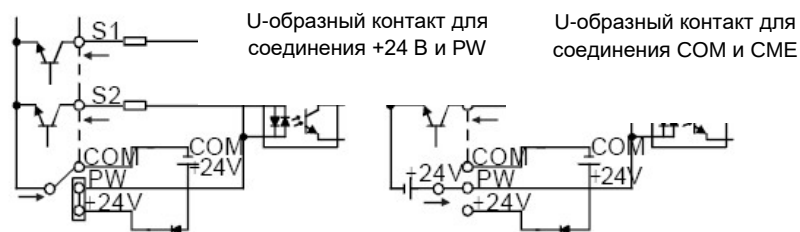
Рис.5-19 NPN режим
