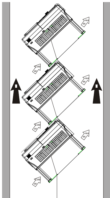
Рис. 4-6 Наклонная установка
