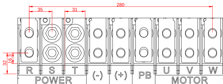
Рис. 4-23 Клеммы силовых цепей 3ф 380В 110–132кВт (единица измерения: мм)
