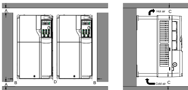
Рис. 4-4 Параллельная установка
