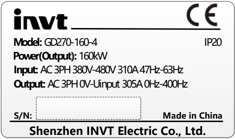
Рис. 3-3 Табличка ПЧ
