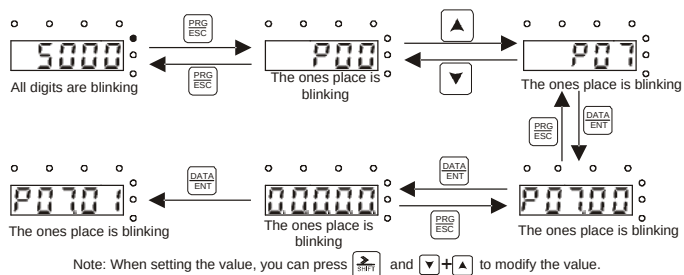
Рис. 5–4 Задание пароля
