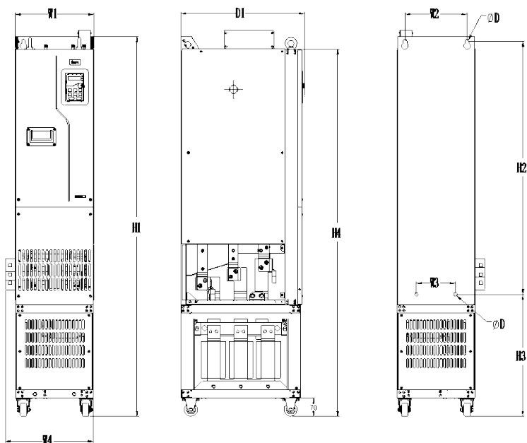
Рис. С-11 Чертеж для напольного монтажа моделей ПЧ 380В 220–500кВт с выходными реакторами
