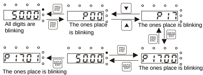
Рис. 5–5 Просмотр параметра
