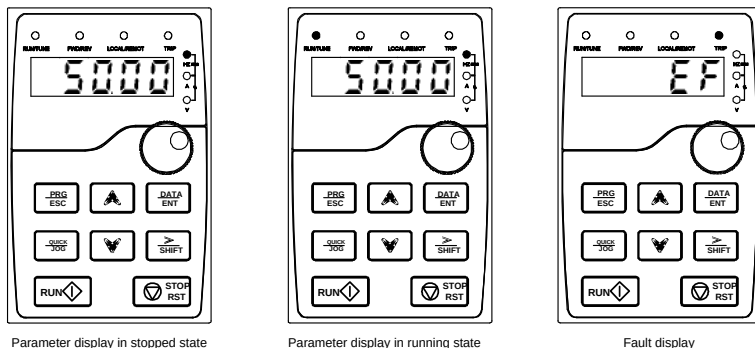
Рис. 5–2 Состояния дисплея
