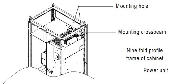
Рис. 4–12 Трехмерный вид крепления GD270-280-4–GD270-500-4 в шкафу
