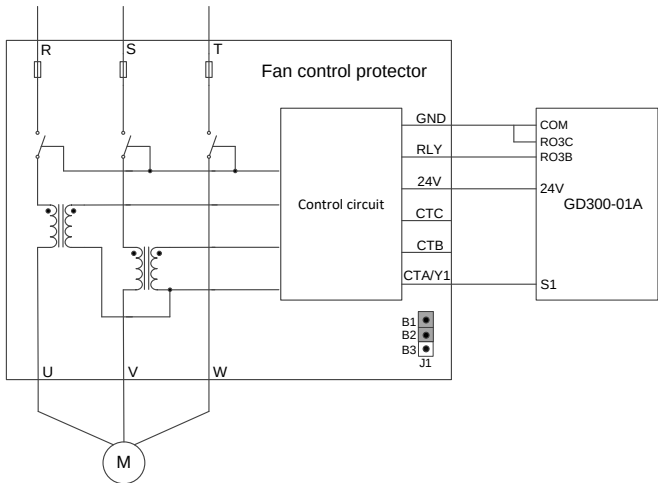
Рис. 8-70 Подключение для MCP100+GD300-01A
