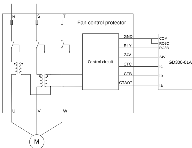
Рис. 8-71 Подключение для MCP120+GD300-01A
