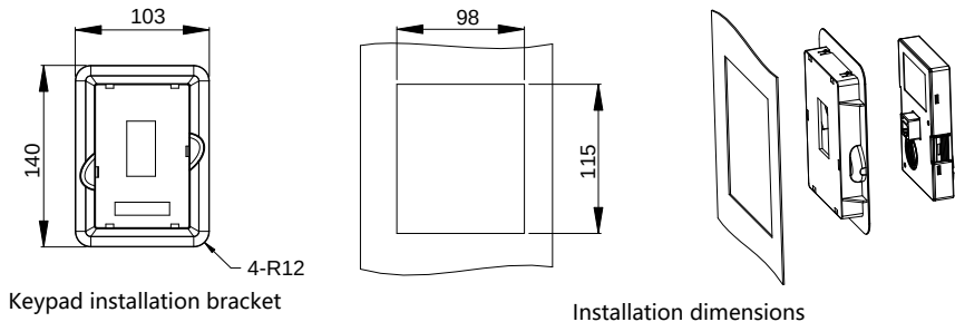
Рис. 8-3 Кронштейн для установки ЖК-панели управления на дверь шкафа
