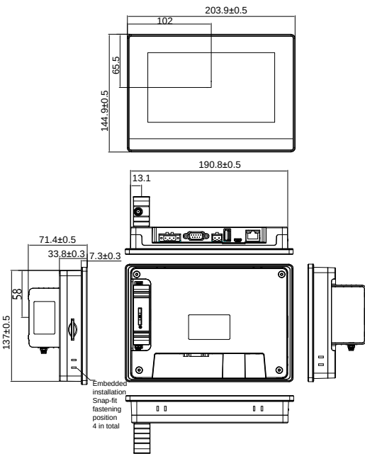
Рис. 8-64 Установочные размеры сенсорного экрана (единица измерения: мм)
