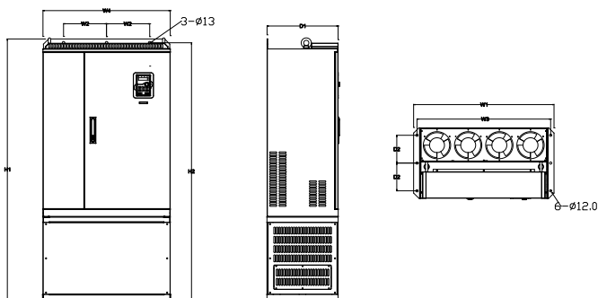
Рис. 7-7 Размеры для напольного монтажа 220кВт–315кВт
