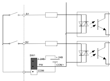
Рисунок 2.5 Внутреннее питание (режим NPN)
