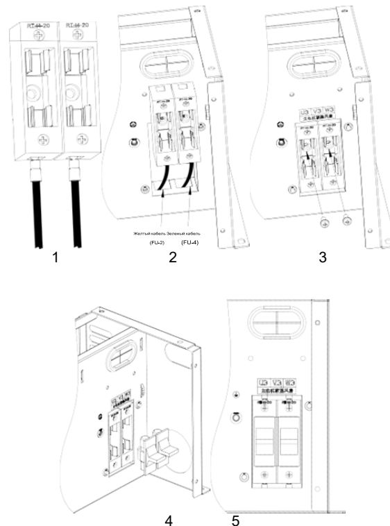
Рисунок В.2 Схема установки подставки для предохранителей
