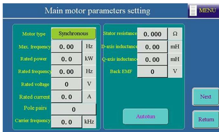
Рисунок 4.10 Интерфейс настройки параметров главного (синхронного) двигателя
