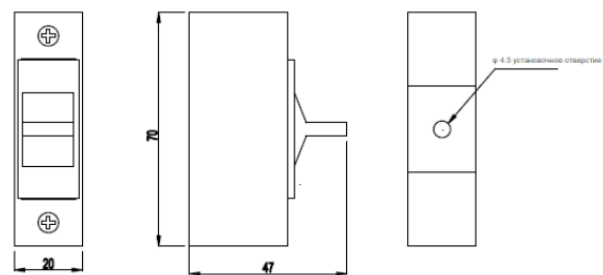
Рисунок В.5 Размер основания предохранителя (единица измерения: мм)
