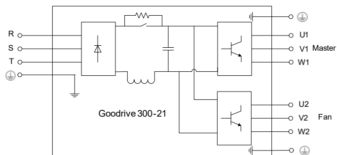
Рисунок 2.1 Схема подключения главной цепи
