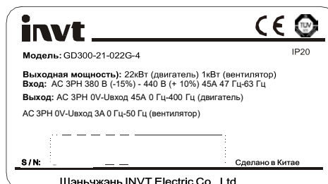
Рисунок 1.1 Паспортная табличка изделия
