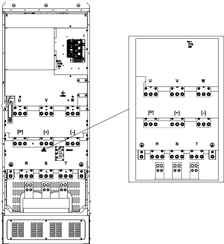
Рис 4.14 Клеммы силовых цепей ПЧ 355G/400P–500G
