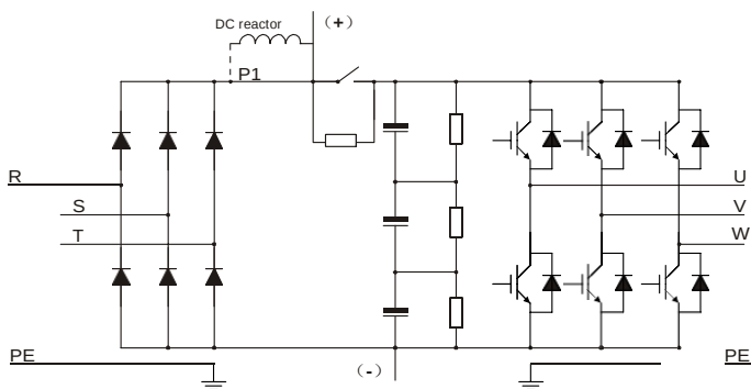
Рис 3.4 Схема силовой цепи ( от 132G/160P до 500G)
