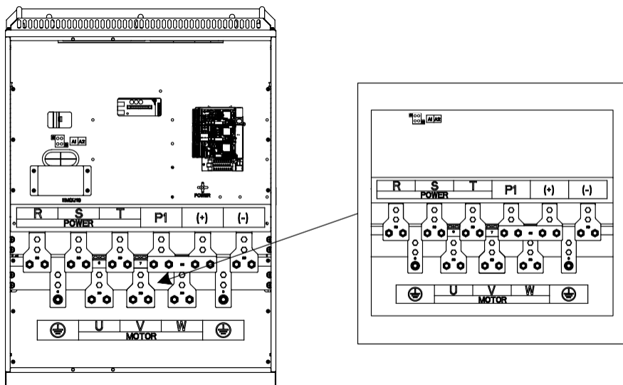
Рис 4.13 Клеммы силовых цепей ПЧ 220G/250P–315G/355P
