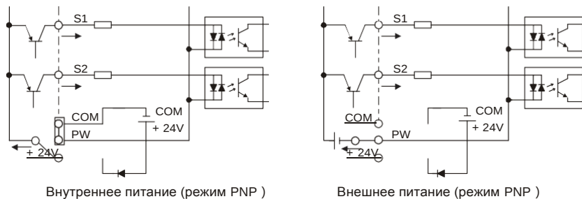
Рис 4.21 PNP режим
