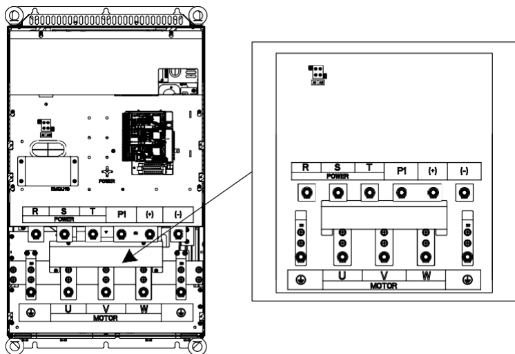
Рис 4.12 Клеммы силовых цепей ПЧ 132G/160P–200G/220P
