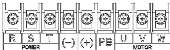
Рис 4.11 Клеммы силовых цепей ПЧ 045G/055P–110G/0132P (дополнительный встроенный тормозной модуль обозначен PB).
