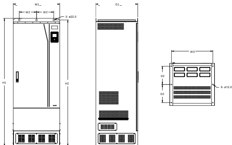
Fig 0.20 Схема для напольного монтажа ПЧ напряжением 660 В, от 400 до 630 кВт Таблица С.6. Установочные размеры ПЧ напольного монтажа 660 В (единица измерения: мм))
