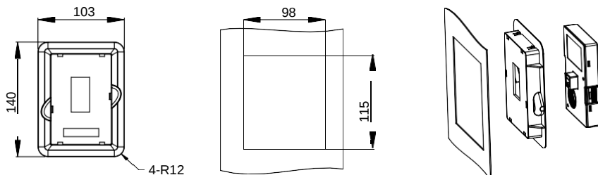
Установочные размеры
