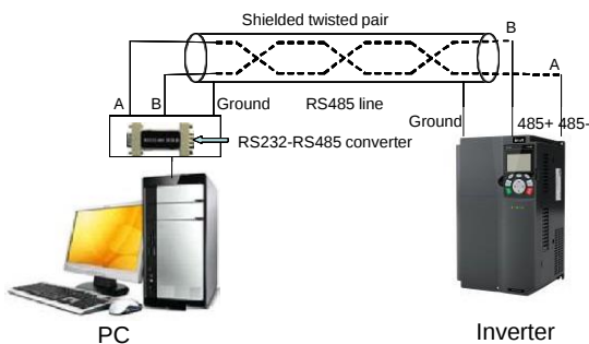
Рис 9.1 Подключение RS485 к одному ПЧ
