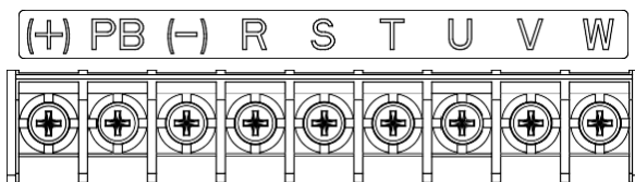
Рис 4.9 Клеммы силовых цепей ПЧ 022G/030P и ниже
