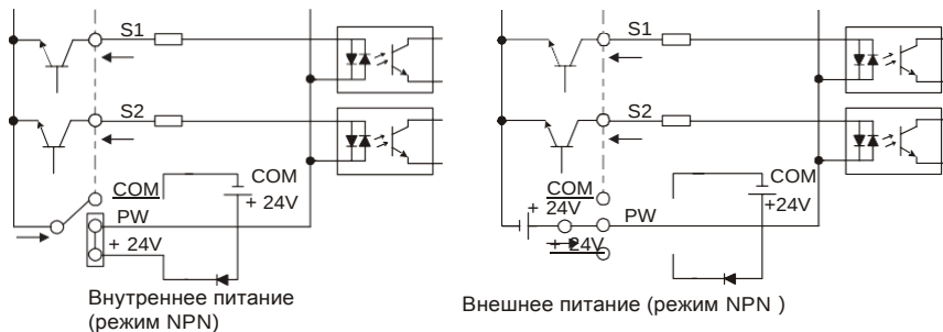
Рис 4.20 NPN режим
