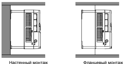
Рис 4.2 Способы установки
