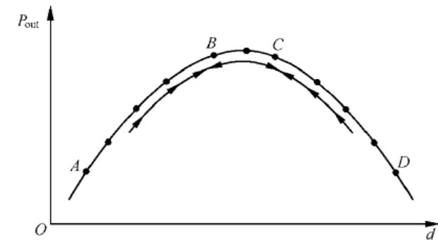
最大功率点跟踪控制原理 MPPT control principle
