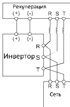
Рисунок 4.9. Подключение блока рекуперации
