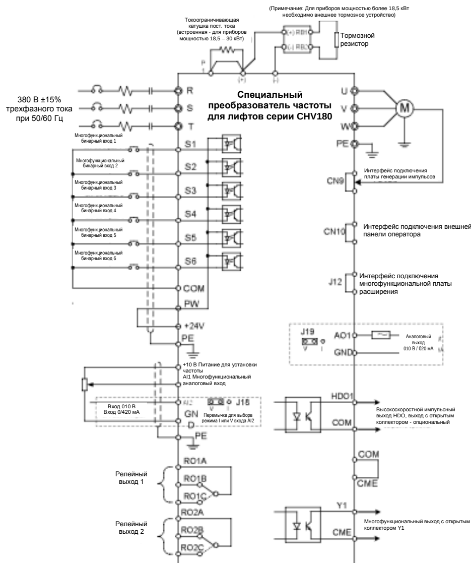
Рисунок 4.6 Схема подключения
