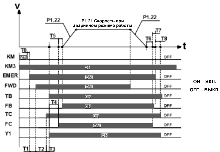
Рисунок А.7 Схема временной последовательности аварийного режима работы
