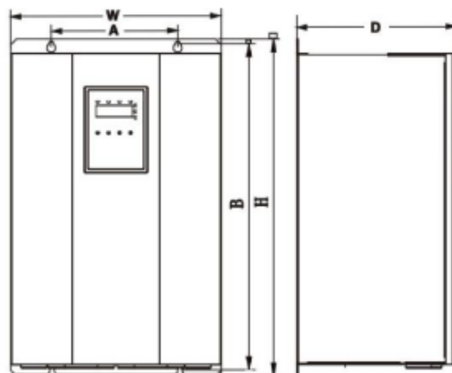
Рисунок В.1 Габаритные размеры (приборы мощностью 15 кВт и менее)
