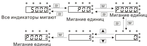
Рис.4-4 Схемы задания пароля
