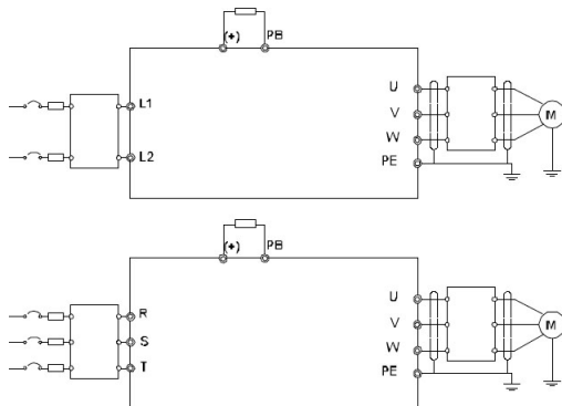
Схема3-3 Подключение силовых цепей
