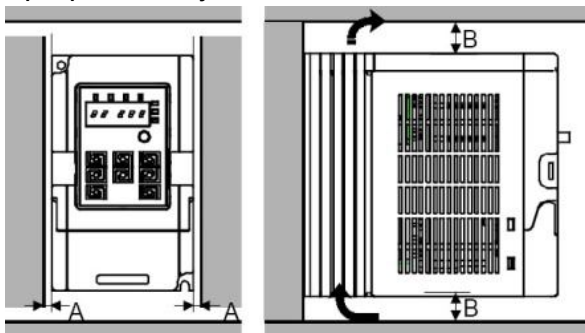
Рис. 3-2 Место установки
