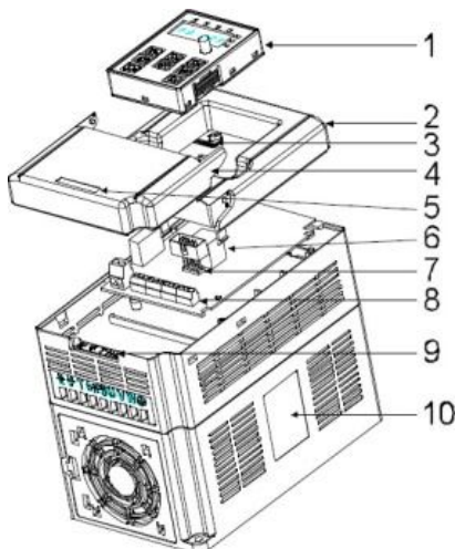
Рис. 2-3 Внешний вид ПЧ
