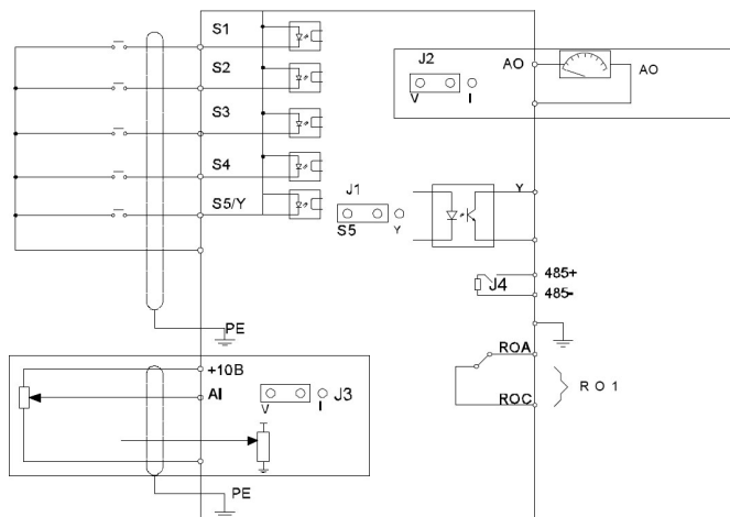
Рис.3-5 Схема подключения цепей управления
