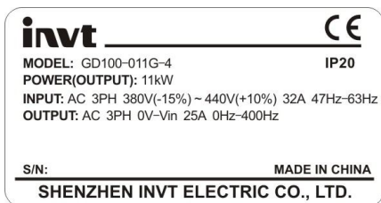
Рис.2-1 Шильдик ПЧ
