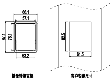
键盘转接支架
