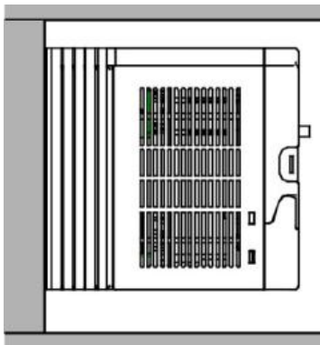
Рис.3-1 Установка ПЧ
