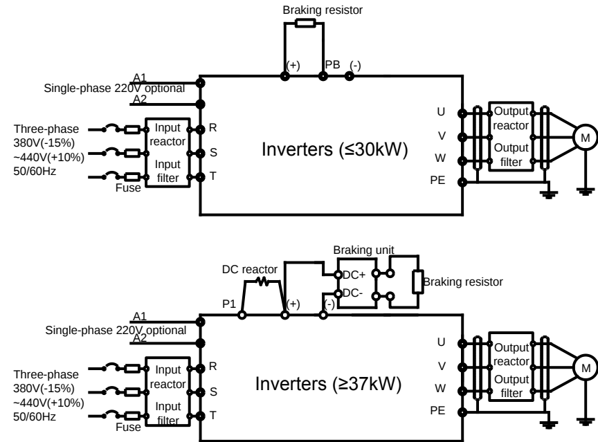
Рис. 3-1 Схема подключения силовых цепей
