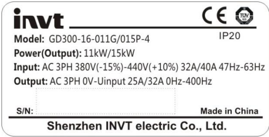
Рис. 2-1 Шильдик инвертора
