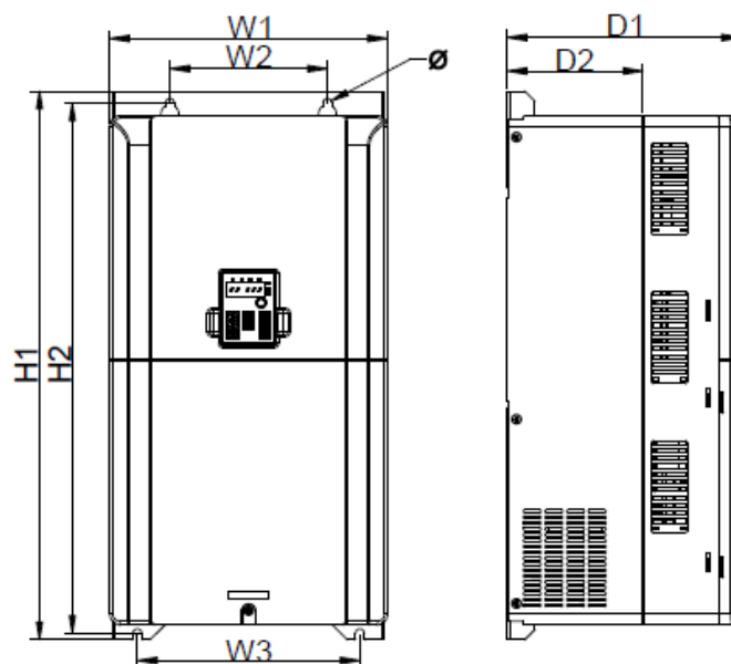
Рис. 4.8 Настенный монтаж 4 – 37 кВт
